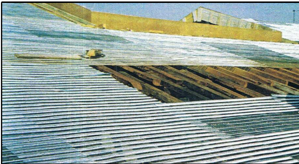
Rehabilitación de cubierta conservando la estructura de madera.
