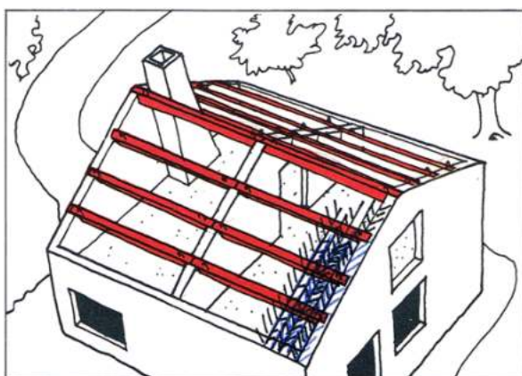
correas paralelas a la cumbrera
