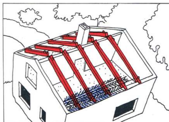
correas perpendiculares a la cumbrera
